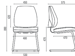
38007 S Aproximação Média
