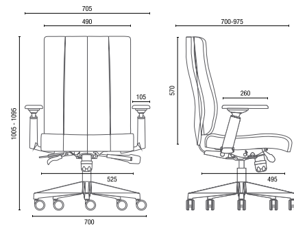
20.502 Diretor Giratória Braços 4D
