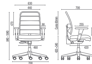
16503 SRE Executiva Giratória
