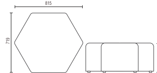
36635 Hexagonal Regular Baixo 350mm
