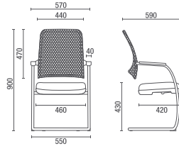
16006 S Executiva Aproximação
