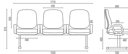
4005 Diretor Longarina Larguras com Braço Duplo: 2L – 1140mm 3L – 1710mm 4L – 2280mm 5L – 2850mm
