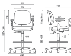
4123 SRE Executiva Caixa
