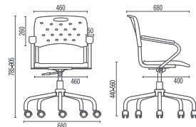
35004 Giratória Base Viva
