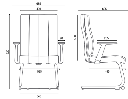
20.506 S Diretor Aproximação Braços fixos em Alumínio
