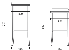
14015 Banqueta Alta / Baixa
