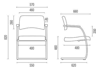
18007 S Secretária Aproximação
