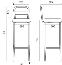
14015 Banqueta Alta com Encosto
