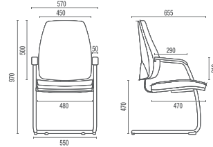
38006 SI Aproximação Alta com Braços Integrados
