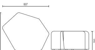
36350 Hexagonal Irregular Baixo 350mm
