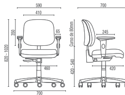
4103 SRE Executiva Giratória
