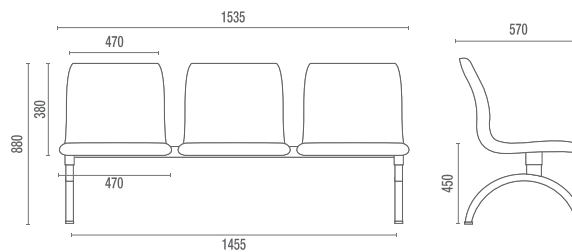
18010 Longarina Larguras sem Braço: 2L – 1000mm 4L – 2070mm 5L – 2605mm Larguras com Braço: 2L – 1080mm 4L – 2110mm 5L – 2625mm
