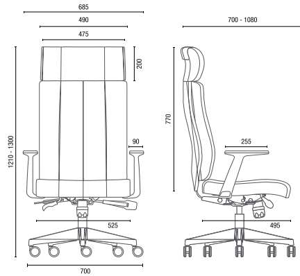
20.501 Presidente Giratória Braços fixos em Alumínio
