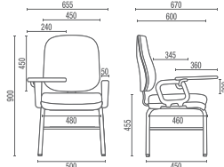
4006 PUE Diretor Universitária
