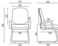
4006 S Diretor Aproximação
