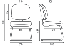
4107 S Executiva Aproximação
