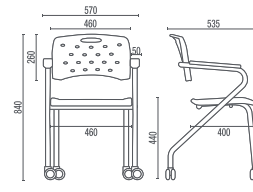
35007 Z ROD Aproximação com Rodízios
