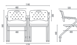
35007 Z Aproximação com Mecanismo de União
