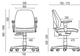
38003 SRE Operacional Média
