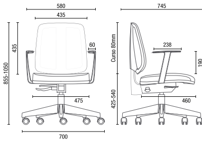
43.103 SRE Executiva Giratória
