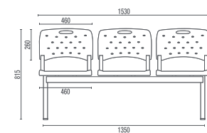
35010 Longarina Larguras sem Braço: 2L - 1026mm 3L - 1530mm 4L - 2052mm 5L - 2578mm
