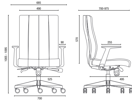
20.502 Diretor Giratória Braços fixos em Alumínio
