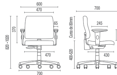
18004 SRE Executiva Giratória
