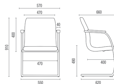
18006 S Diretor Aproximação
