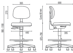
4022 SRE Secretária Caixa
