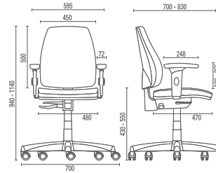
38001 SRE Operacional Alta
