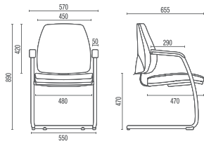
38007 SI Aproximação Média com Braços Integrados
