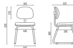
4008 A Secretária Aproximação
