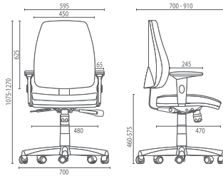
38001 L Presidente Giratória
