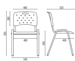
35008 P Aproximação Empilhável
