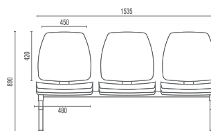
38010 Longarina Média Larguras: 2L - 1010mm 4L - 2070mm 5L - 2600mm
