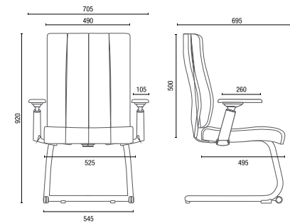
20.506 S Diretor Aproximação Braços 4D
