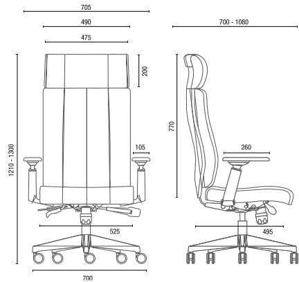
20.501 Presidente Giratória Braços 4D
