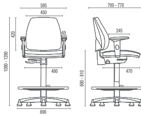
38022 SRE Caixa Média
