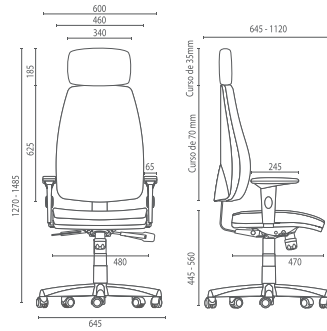
38001 AC Presidente Giratória
